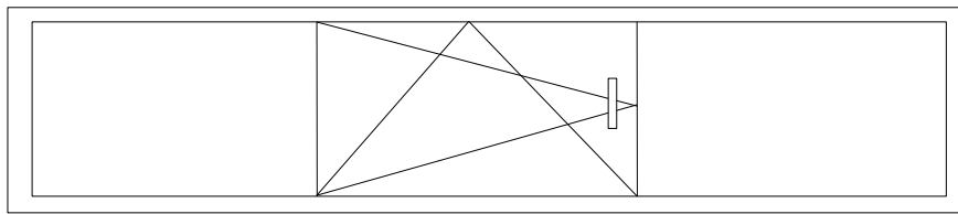
Окно: 2080ммx800мм (h)- 3 шт.
