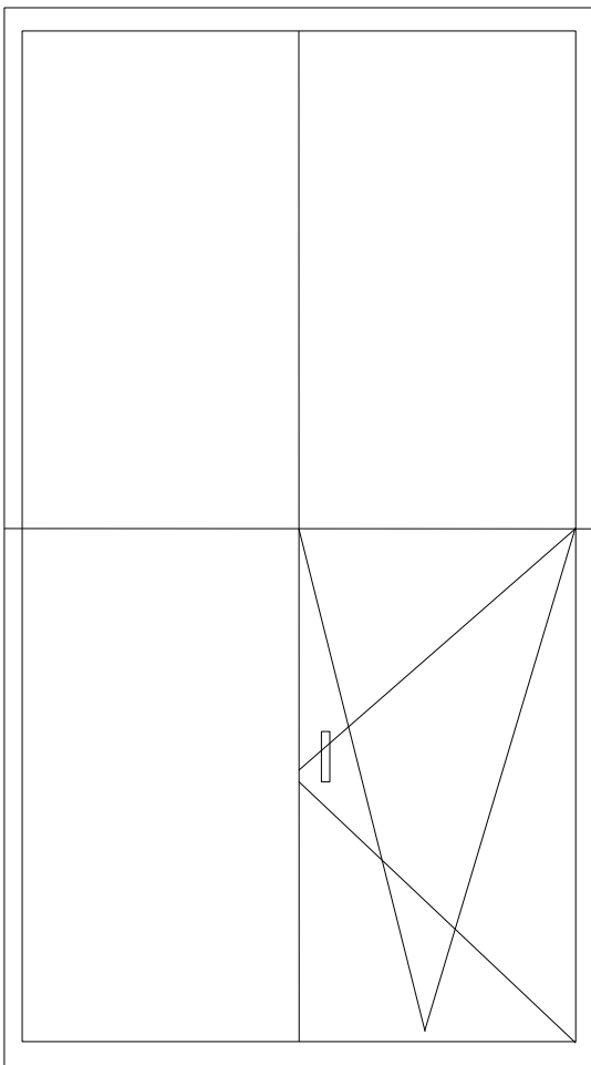
Окно:1370мм x 2230 мм (h) – 9шт.
