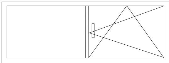
Окно: 1250мм x 650мм (h)- 3 шт.
