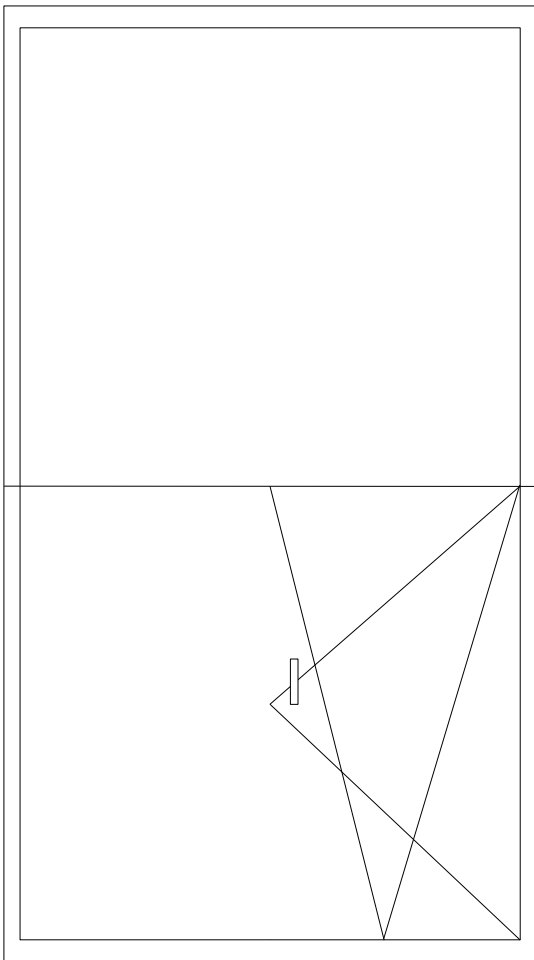
Окно: 2050мм x 650мм (h) - 3 шт.
