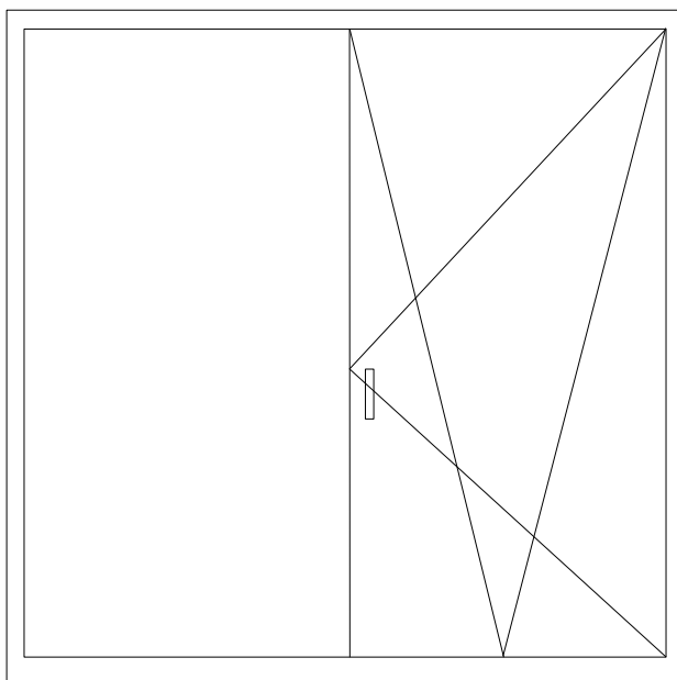
Окно: 1330мм x 1370 мм (h) – 12 шт.
