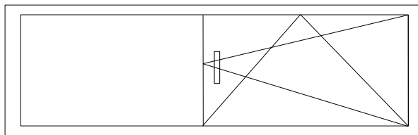
Окно: 1330мм x 750мм (h) - 3 шт.
