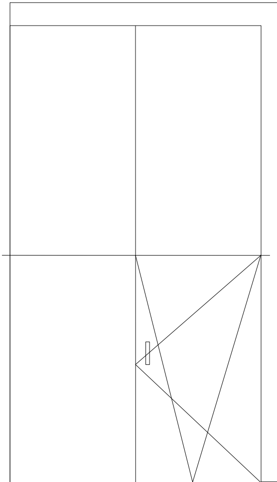
Окно: 2040x650 мм (h)- 4 шт.
