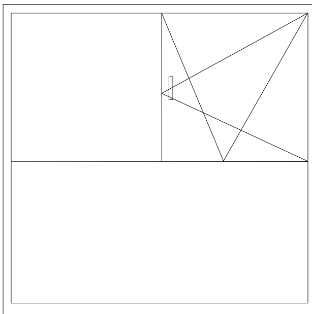
Окно: 1270мм x 1310 мм (h) – 4 шт.
