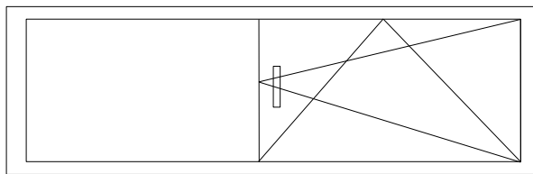
Окно: 1270мм x 570мм (h) - 3 шт.
