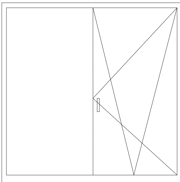
Окно: 1270мм x 1300 мм (h) – 12 шт.
