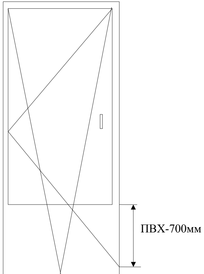
Дверь: 870мм x 2160 мм (h) -4 шт.
