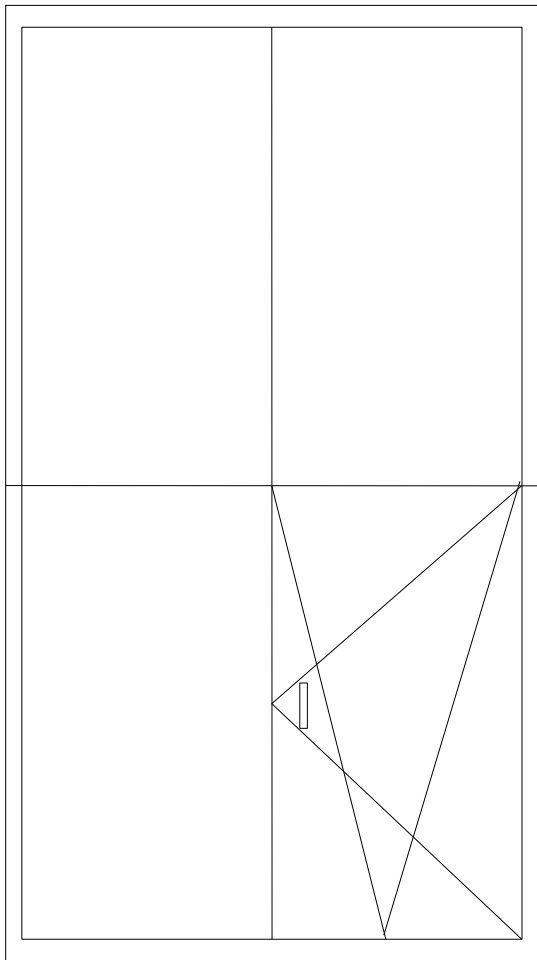
Окно: 1250мм x 2180 мм (h) -4 шт.
