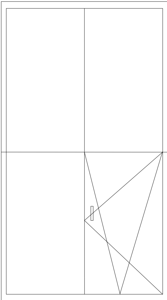
Окно:1230мм x 2200 мм (h) – 16шт.
