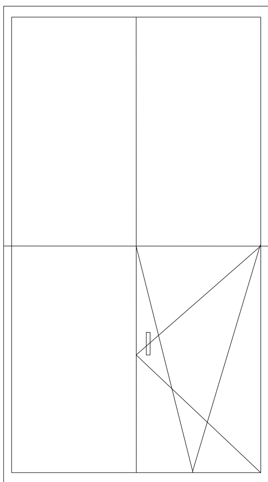
Окно: 2050мм x 620мм (h) - 4 шт.
